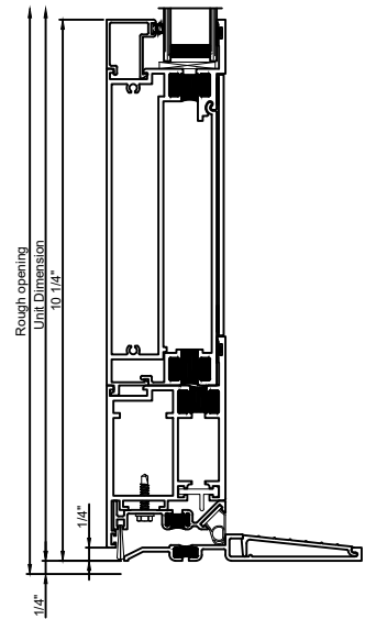
ADA Sill 10"
