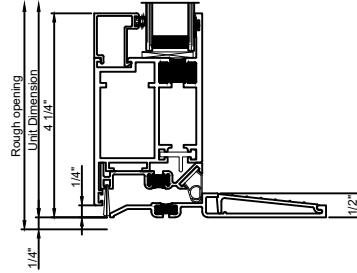
ADA Sill
