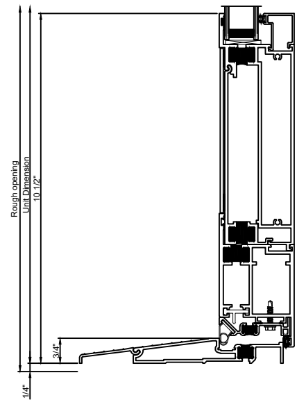
ADA Sill 10"
